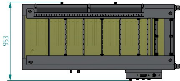
VISTA PLANTA
